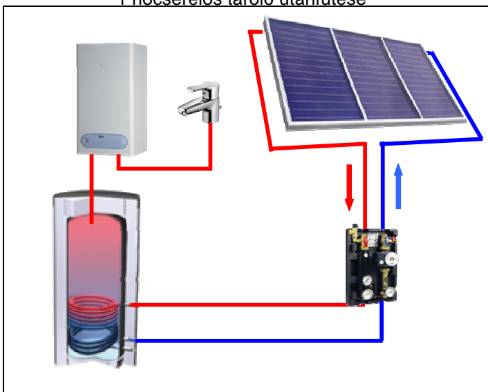
1 hőcserélős tároló utánfűtése
