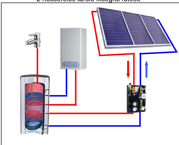
2 hőcserélős tároló kiegészítő fűtése
