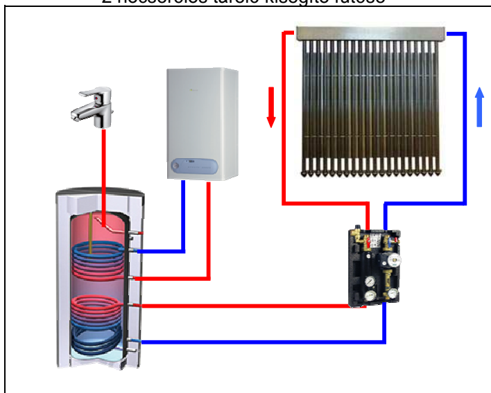
2 hőcserélős tároló kiegészítő fűtése
