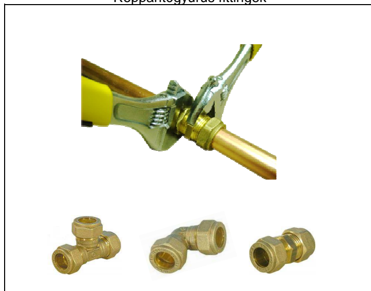
Roppantógyűrűs fittingek
